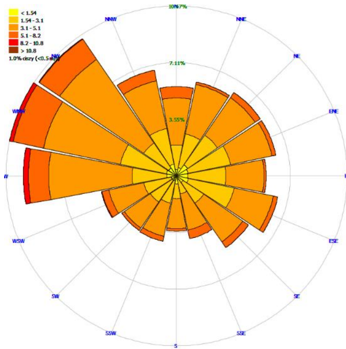
Rysunek 20 Rozkład kierunków i prędkości wiatru w okresie letnim w Radomiu, w 2018 roku
