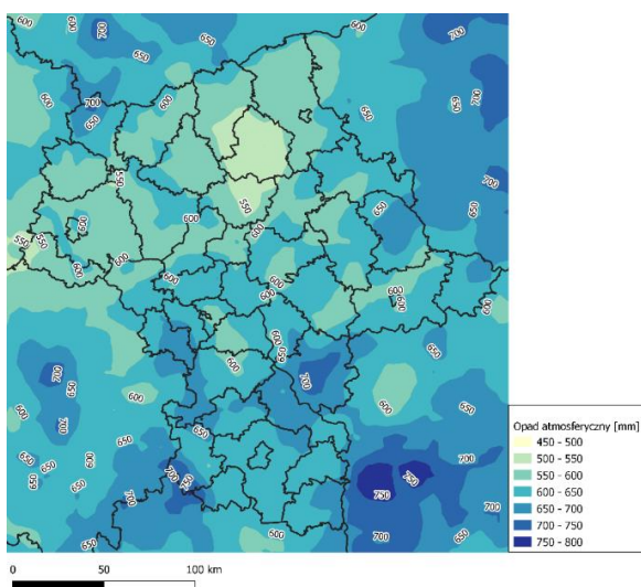
Rysunek 40 Przestrzenny rozkład rocznych sum opadów atmosferycznych [mm], wyznaczonych przez model WRF/CALMET, w województwie mazowieckim, w 2018 roku
