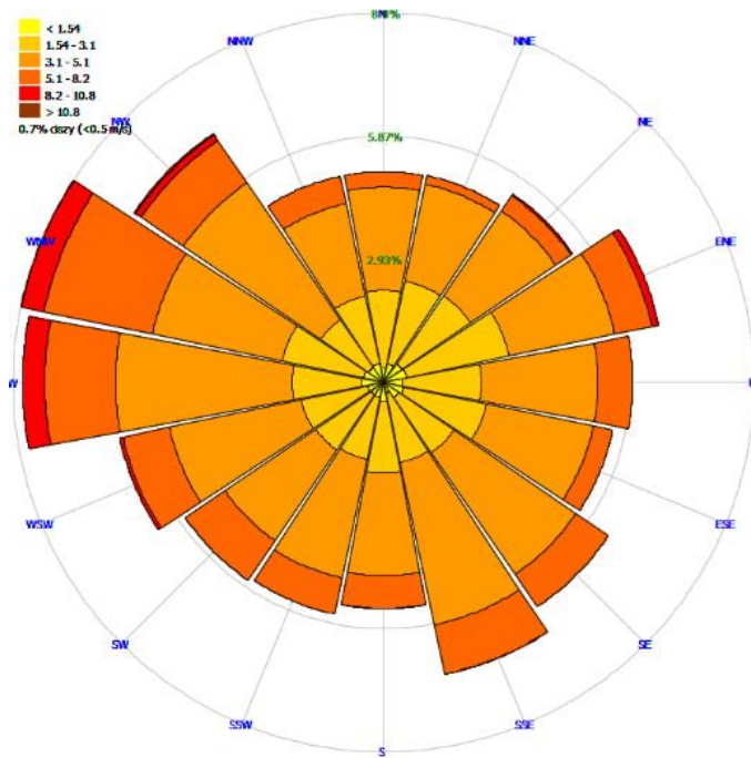
Rysunek 32 Rozkład kierunków i prędkości wiatru w Radomiu w całym w 2018 roku
