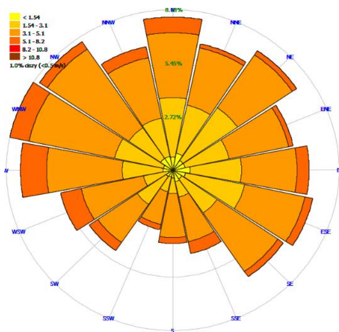
Rysunek 18 Rozkład kierunków i prędkości wiatru w okresie letnim w Warszawie, w 2018 roku
