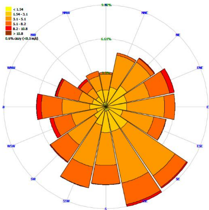
Rysunek 27 Rozkład kierunków i prędkości wiatru w Ostrołęce w okresie zimowym w 2018 roku
