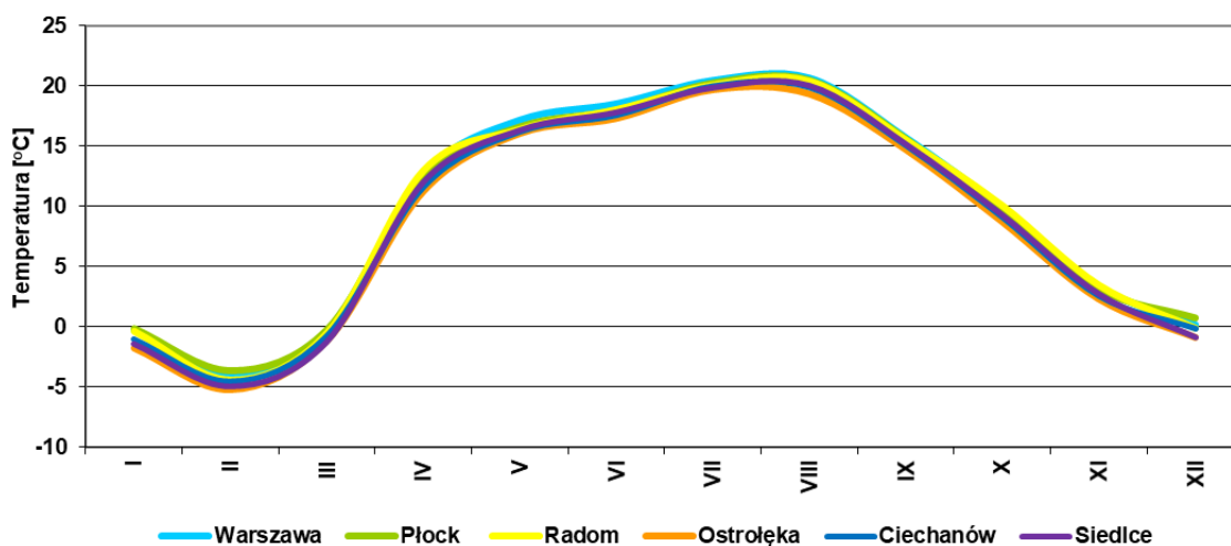
Rysunek 37 Przebiegi średnich miesięcznych temperatur [°C] powietrza wyznaczone przez model WRF/CALMET w miejscowościach województwa mazowieckiego w 2018 roku
