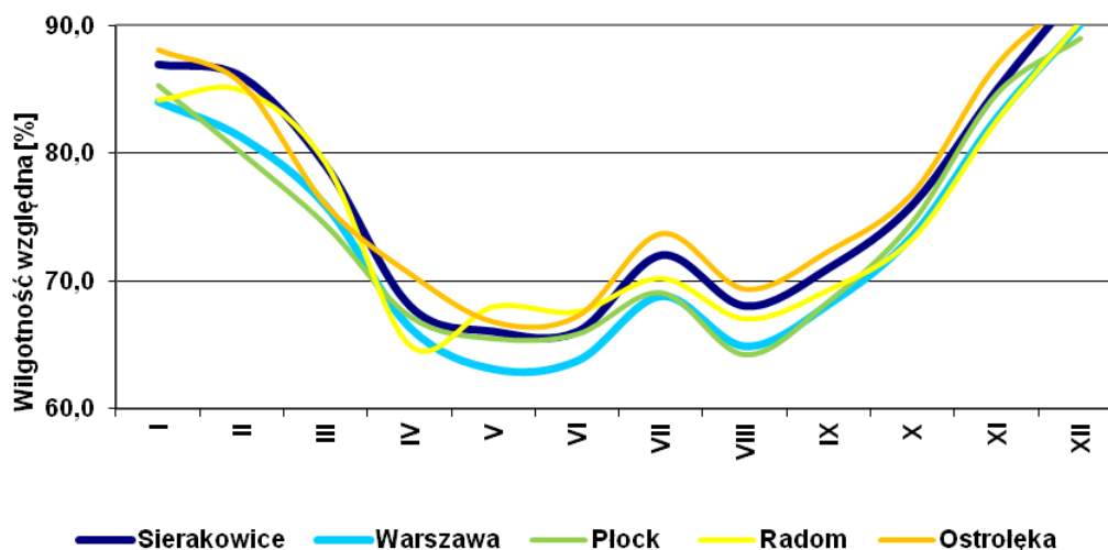
Rysunek 43 Przebiegi wilgotności względnej powietrza [%] w wybranych miejscowościach województwa mazowieckiego w 2018 roku
