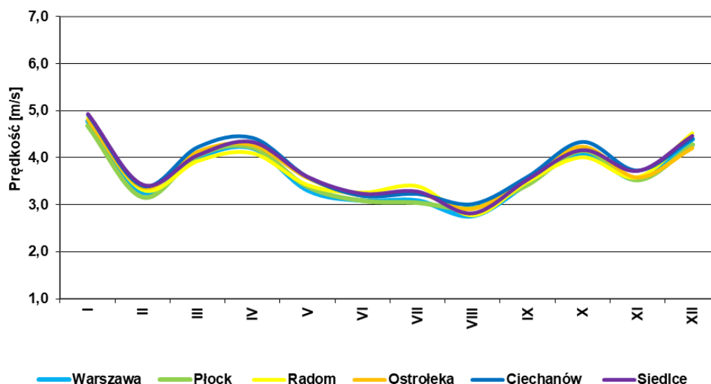
Rysunek 16 Średnie miesięczne prędkości wiatru [m/s] wyznaczone przez model WRF/CALMET dla wybranych miejscowości w województwie mazowieckim, w 2018 roku
