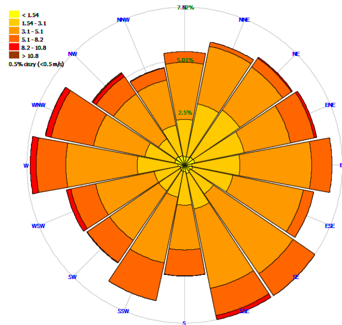
Rysunek 34 Rozkład kierunków i prędkości wiatru w Ciechanowie w całym w 2018 roku
