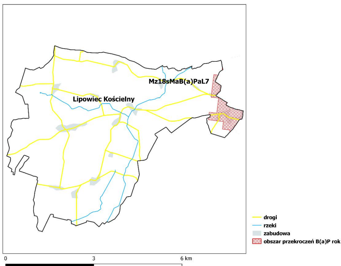
Rysunek 170 Obszar przekroczeń poziomu docelowego średniorocznego benzo(a)pirenu Mz18sMaB(a)PaL7 w gminie wiejskiej Lipowiec Kościelny w 2018 roku
