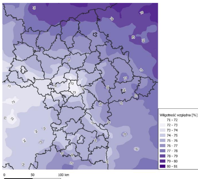
Rysunek 42 Przestrzenny rozkład średniej rocznej wilgotności względnej powietrza [%], wyznaczonej przez model WRF/CALMET, w województwie mazowieckim, w 2018 roku
