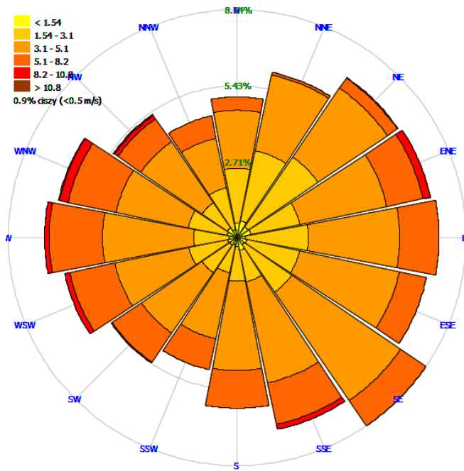
Rysunek 34 Rozkład kierunków i prędkości wiatru w Ciechanowie w całym w 2018 roku
