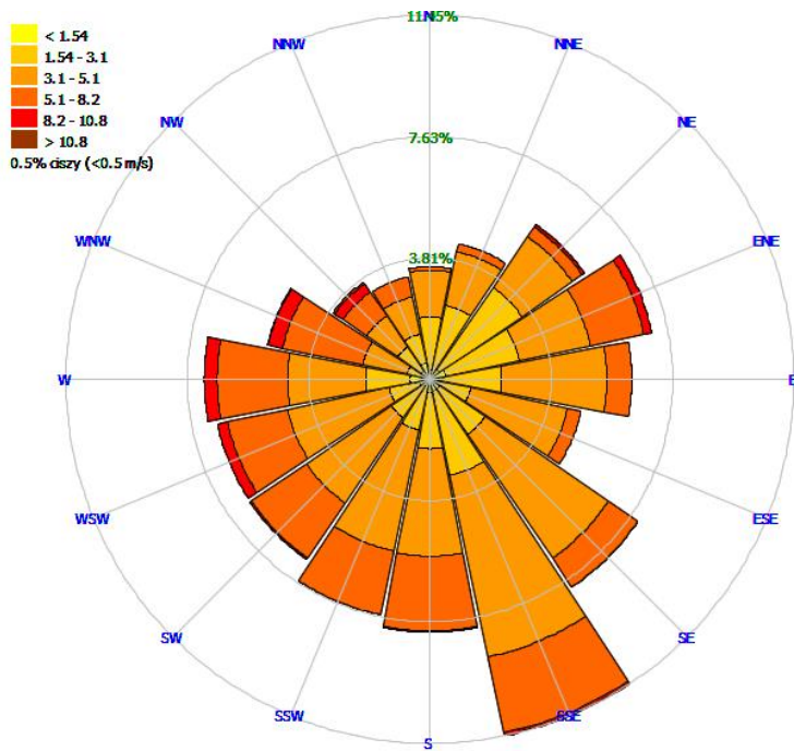
Rysunek 24 Rozkład kierunków i prędkości wiatru w Warszawie w okresie zimowym w 2018 roku
