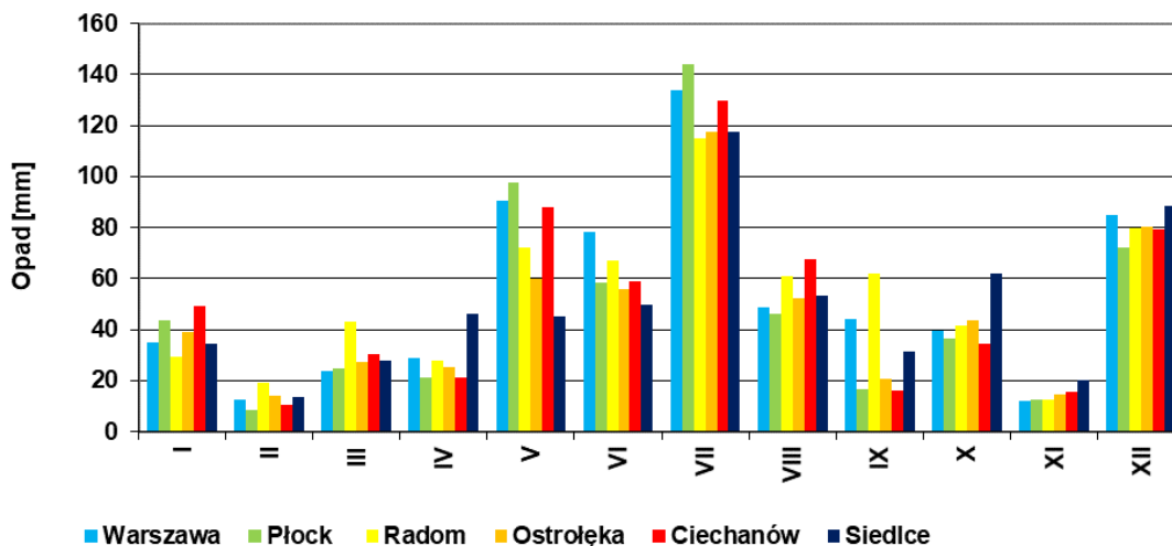
Rysunek 41 Miesięczne sumy opadów atmosferycznych wyznaczone przez modele WRF/CALMET w miejscowościach województwa mazowieckiego w 2018 roku
