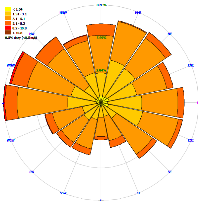
Rysunek 23 Rozkład kierunków i prędkości wiatru w okresie letnim w Siedlcach, w 2018 roku
