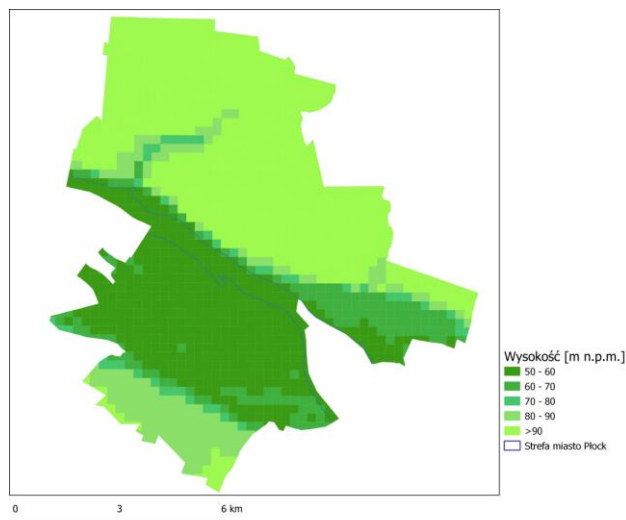
Rysunek 419 Rzeźba terenu w strefie miasto Płock
