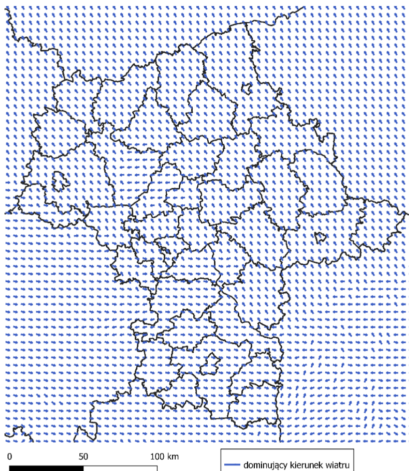
Rysunek 17 Dominujący kierunek wiatru wyznaczony przez model WRF/CALMET dla województwa mazowieckiego, w 2018 roku
