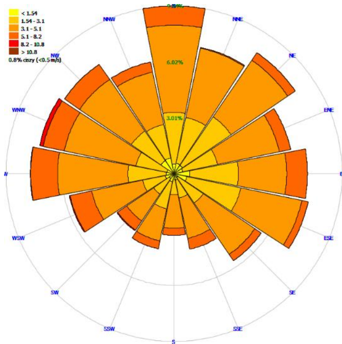
Rysunek 21 Rozkład kierunków i prędkości wiatru w okresie letnim w Ostrołęce, w 2018 roku
