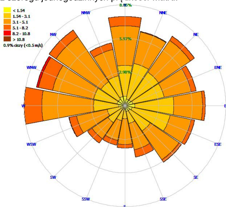
Rysunek 18 Rozkład kierunków i prędkości wiatru w okresie letnim w Warszawie, w 2018 roku
