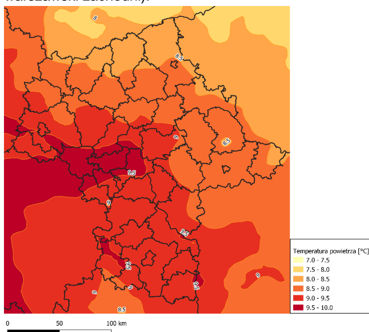
Rysunek 36 Przestrzenny rozkład średnich rocznych temperatur [°C] powietrza wyznaczonych przez WRF/CALMET w województwie mazowieckim, w 2018 roku
