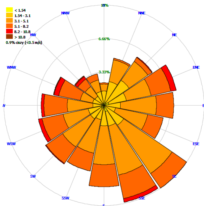
Rysunek 28 Rozkład kierunków i prędkości wiatru w Ciechanowie w okresie zimowym w 2018 roku
