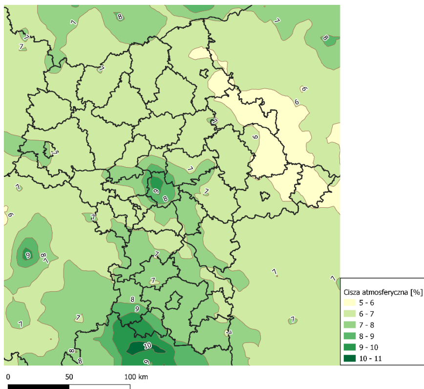
Rysunek 14 Przestrzenny rozkład częstości występowania cisz atmosferycznych (prędkość mniejsza od 1,5 m/s) [%] wyznaczonych przez model WRF/CALMET, w województwie mazowieckim, w 2018 roku
