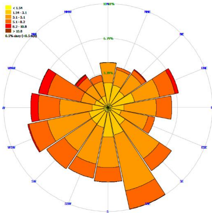
Rysunek 26 Rozkład kierunków i prędkości wiatru w Radomiu w okresie zimowym w 2018 roku
