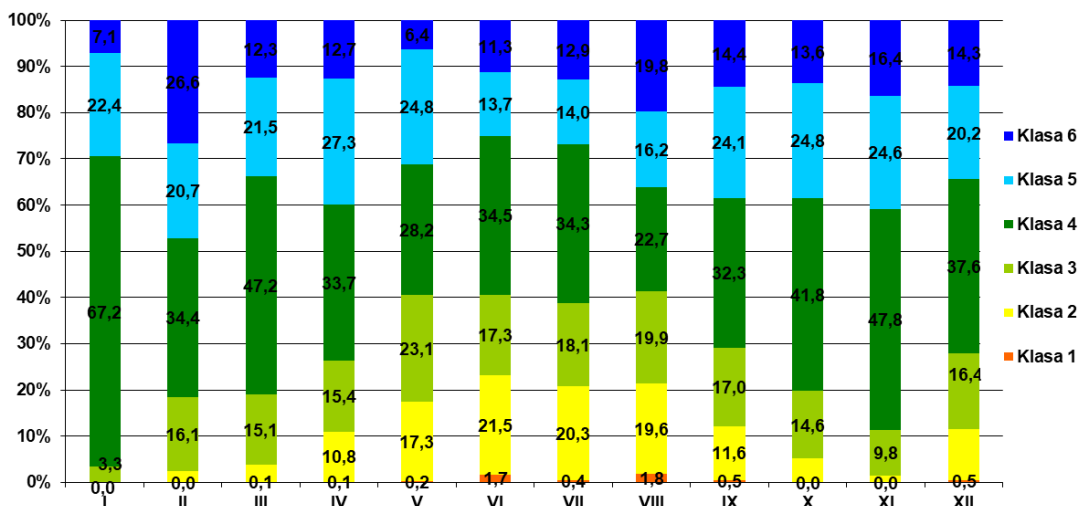
Rysunek 38 Udział procentowy klas równowagi atmosfery Pasquilla wyznaczonych przez model WRF/CALMET w województwie mazowieckim w 2018 roku
