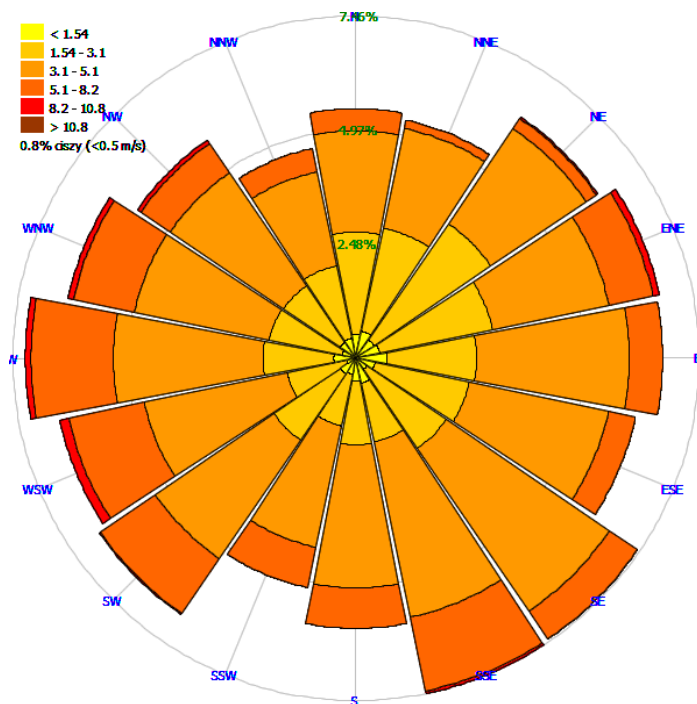
Rysunek 30 Rozkład kierunków i prędkości wiatru w Warszawie w całym w 2018 roku
