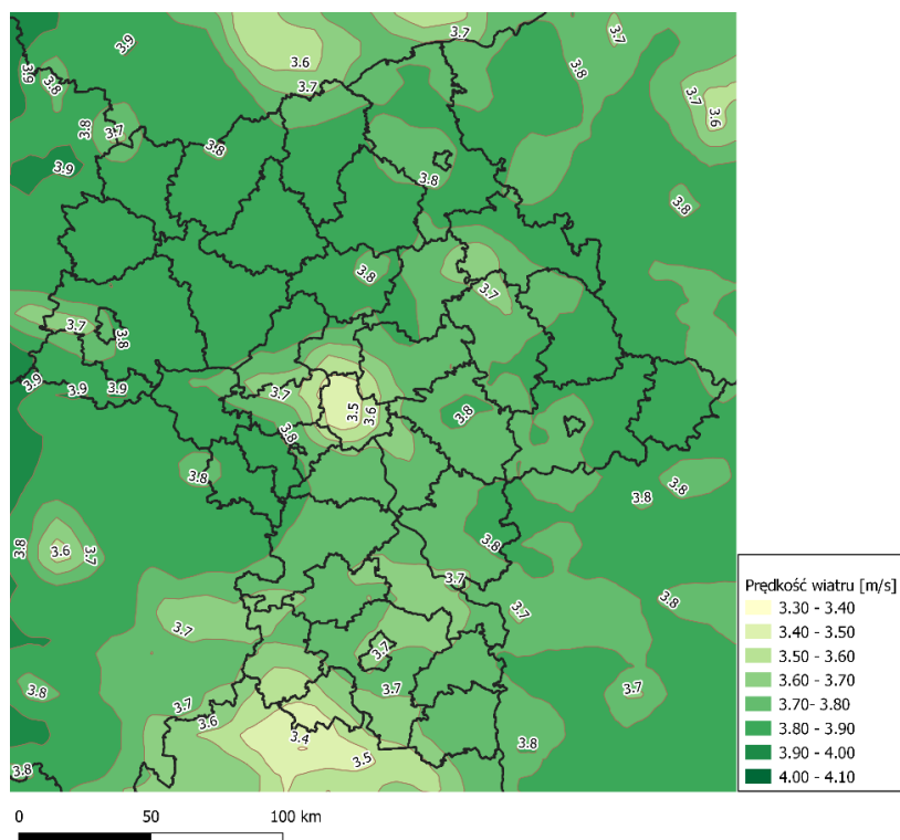
Rysunek 13 Przestrzenny rozkład średnich rocznych prędkości wiatru [m/s] wyznaczonych przez model WRF/CALMET w województwie mazowieckim, w 2018 roku
