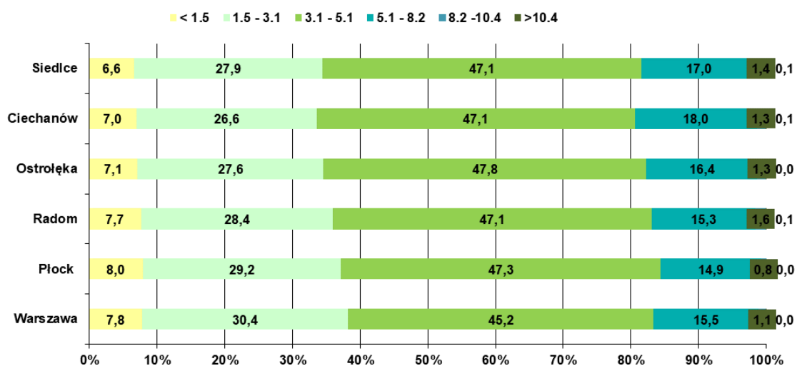
Rysunek 15 Częstość [%] występowania prędkości wiatru [m/s] w określonych przedziałach, w miejscowościach województwa mazowieckiego, w 2018 roku
