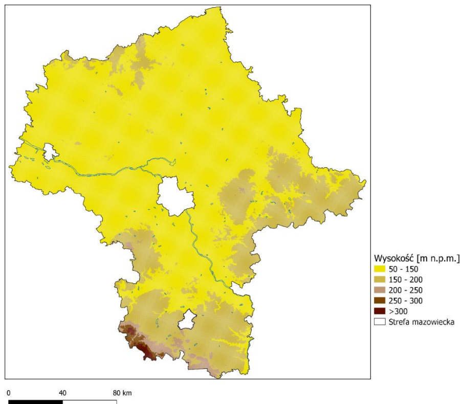
Rysunek 45 Rzeźba terenu strefy mazowieckiej
