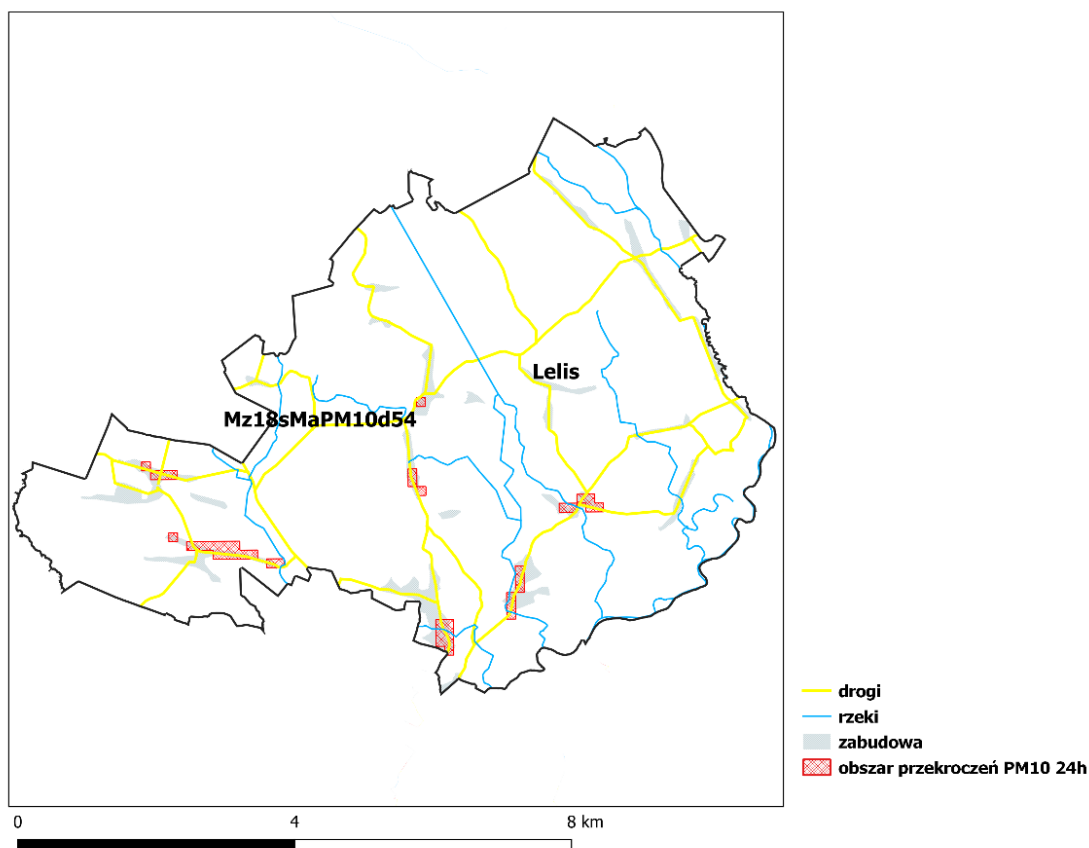
Rysunek 164 Obszar przekroczeń poziomu dopuszczalnego średniodobowego pyłu zawieszonego PM10 Mz18sMaPM10d54 w gminie wiejskiej Lelis w 2018 roku
