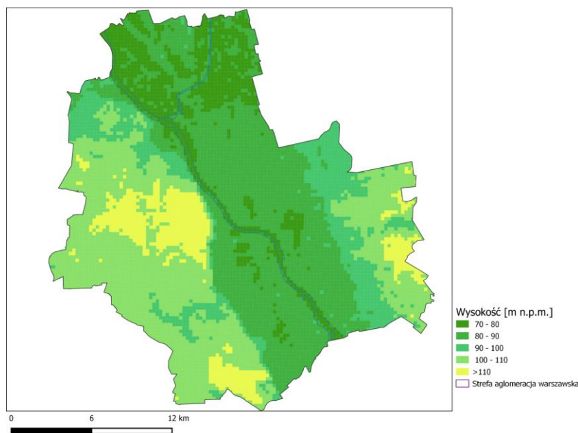
Rysunek 411 Rzeźba terenu w strefie aglomeracja warszawska
