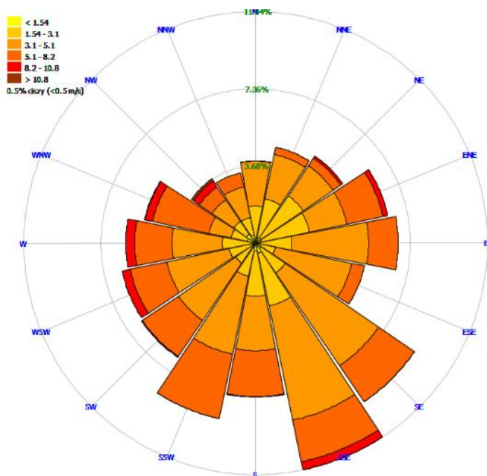
Rysunek 29 Rozkład kierunków i prędkości wiatru w Siedlcach w okresie zimowym w 2018 roku
