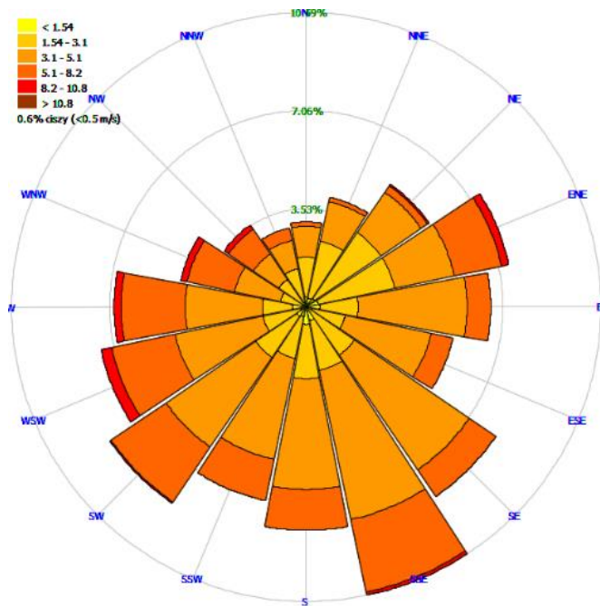
Rysunek 24 Rozkład kierunków i prędkości wiatru w Warszawie w okresie zimowym w 2018 roku
