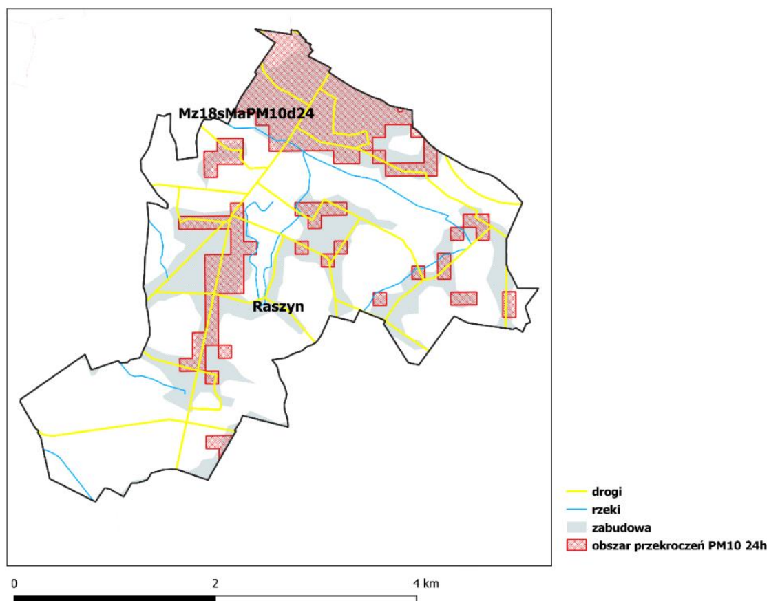
Rysunek 293 Obszar przekroczeń poziomu dopuszczalnego średniodobowego pyłu zawieszonego PM10 Mz18sMaPM10d24 w gminie wiejskiej Raszyn w 2018 roku
