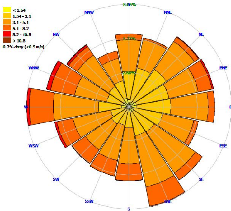
Rysunek 30 Rozkład kierunków i prędkości wiatru w Warszawie w całym w 2018 roku
