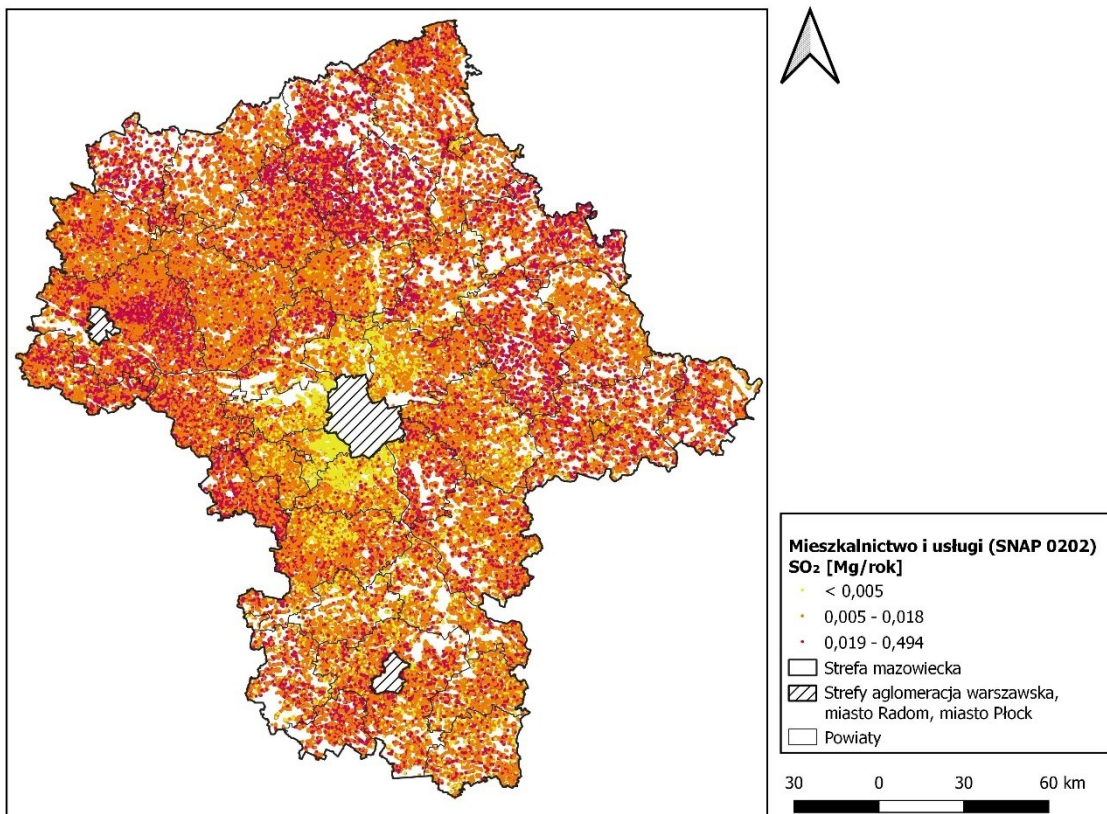
Rysunek 4 Rozmieszczenie oraz ładunki emisji dwutlenku siarki w sektorze mieszkalnictwo (SNAP 0202) w strefie mazowieckiej w 2021 r.
