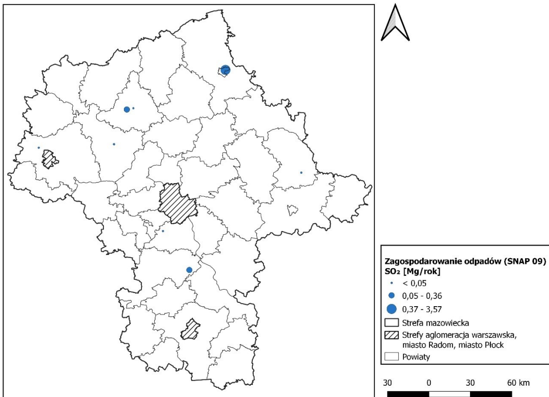
Rysunek 11 Rozmieszczenie oraz ładunki emisji dwutlenku siarki z zagospodarowania odpadów (SNAP 09) w strefie mazowieckiej w 2021 r.
