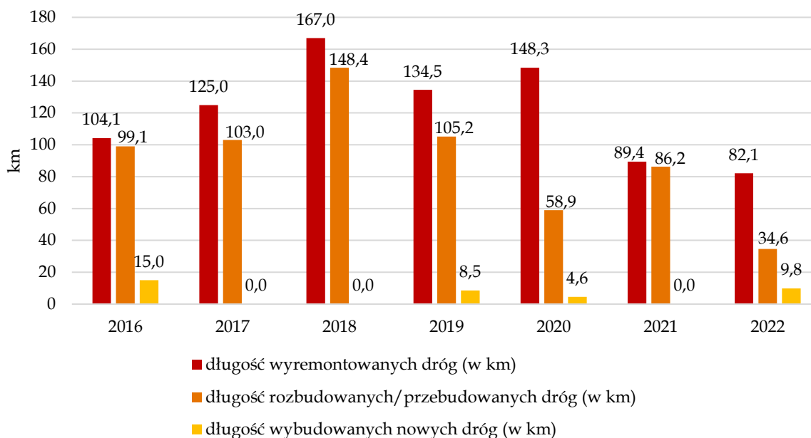
Wykres 3. Podsumowanie inwestycji w ciągu dróg wojewódzkich w latach 2016-2022
