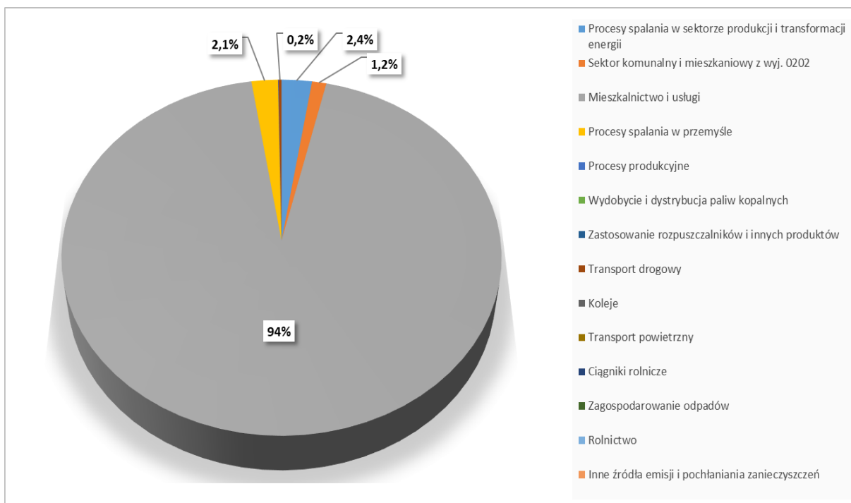
Rysunek 3 Bilans emisji benzo(a)pirenu [%] wg kategorii SNAP ze strefy mazowieckiej w 2018 r.
