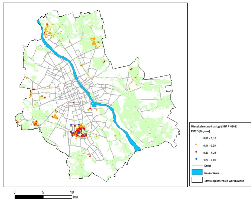
Rysunek 89 Rozmieszczenie oraz ładunki emisji pyłu zawieszonego PM2,5 w mieszkalnictwie i usługach (SNAP 0202) w strefie aglomeracji warszawskiej w 2018 r.
